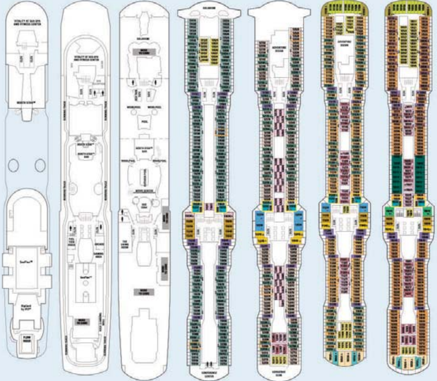
ΚΑΤΑΣΤΡΩΜΑ 16
